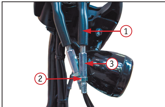
Фото 3. Регулировка троса газа: 1 – защитный колпачок; 2 – стопорная гайка; 3 – регулировочная гайка
