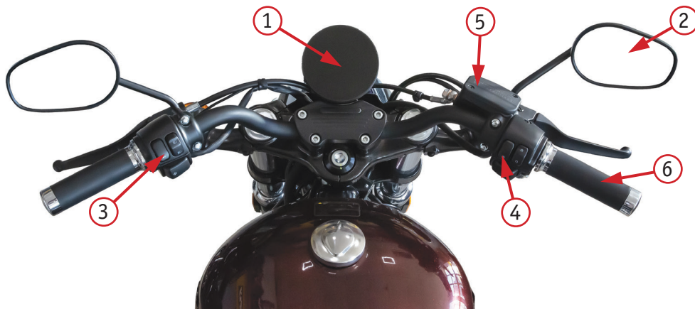
Фото 2.1. Вид руля и органов управления мотоцикла: 1 – приборная панель; 2 – зеркало заднего вида; 3 – левый комбинированный переключатель; 4 – правый комбинированный переключатель; 5 – бачок для тормозной жидкости; 6 – рукоятка газа (акселератор)
