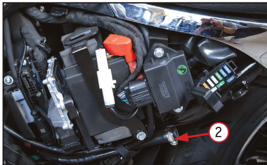
Фото 5.5. Шланг для слива масла с заглушкой - 2
