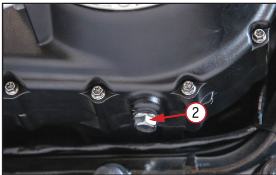
Фото 5.7. Замена масла в коробке передач: 1 – крышка картера; 2 – сливная пробка
