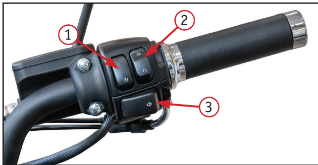
Фото 2.5. Правый комбинированный переключатель: 1 – кнопка электростартера; 2 – переключатель освещения; 3 – кнопка правого указателя поворота
