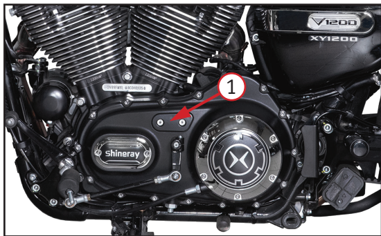
Фото 5.7. Замена масла в коробке передач: 1 – крышка картера; 2 – сливная пробка
