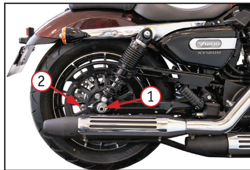
Фото 5.9 Регулировка ремня: 1 - гайка задней оси; 2 - регулировочный болт
