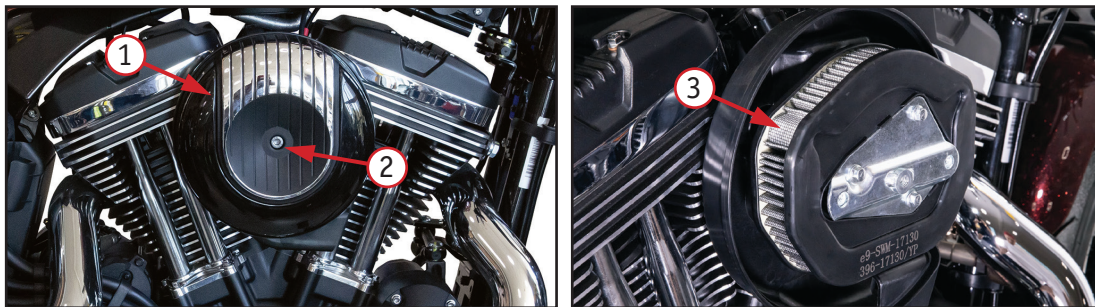
Фото 5.1 Воздушный фильтр: 1 – крышка, 2 – винт крепления; 3 - фильтр
