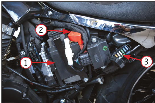
Фото 4.1 Аккумуляторный отсек:
