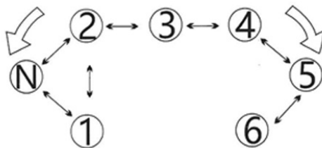
Рисунок 1. Схема переключения передач
