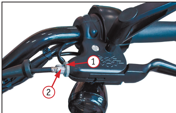
Фото 2.11. Регулировка сцепления: 1 – стопорная гайка; 2 – регулировочный винт
